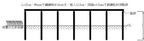
不銹鋼管施工圖
