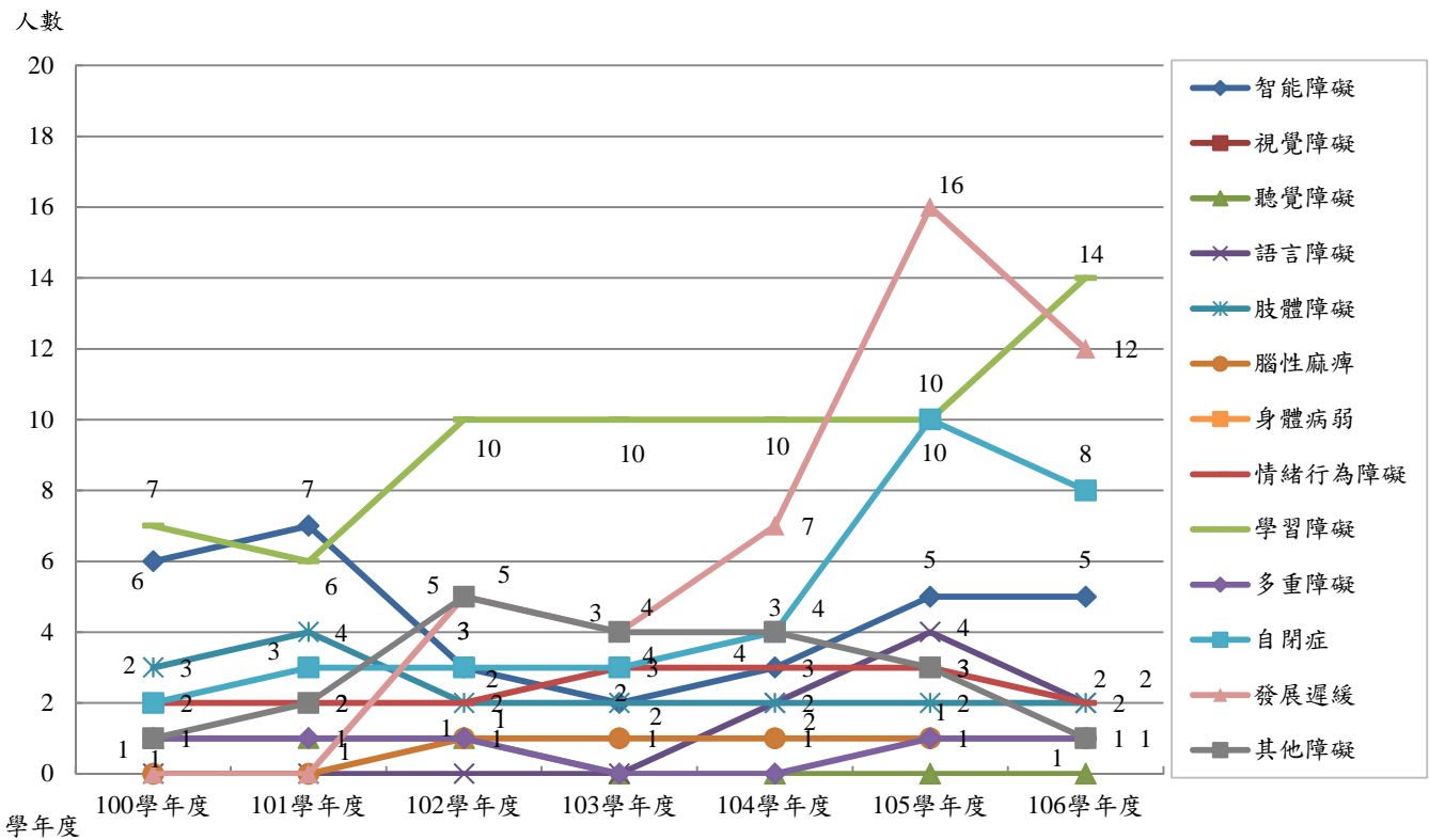
圖1-14：連江縣100至106學年度學前至國中階段各障別學生人數增減趨勢
