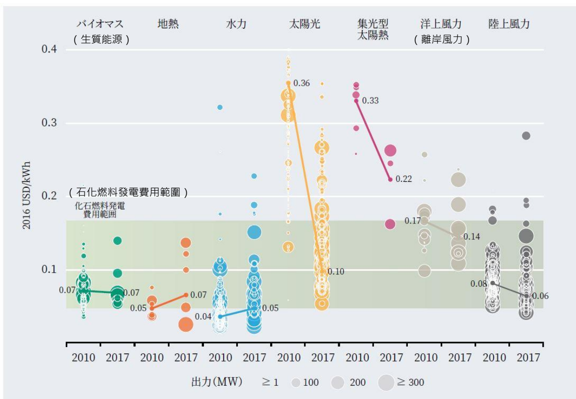
圖 2-4-2 2010 及 2017 年國際各類再生能源發電成本趨勢圖
